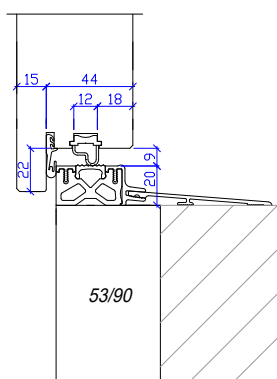
Seuil Hebgo 173 avec 185.W
