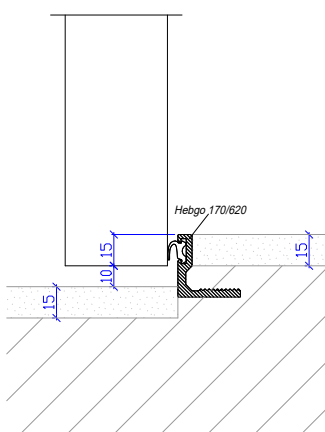
Seuil Hebgo 170
