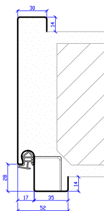
Huisserie UD
