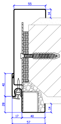
Huisserie ST6.UD
